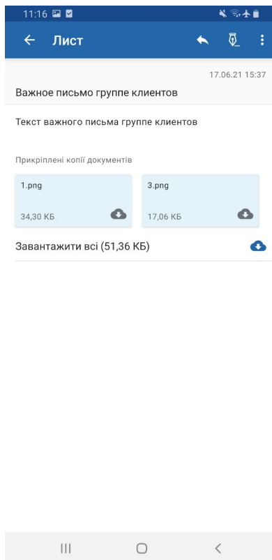
Рис. 8.5. Перегляд листа
