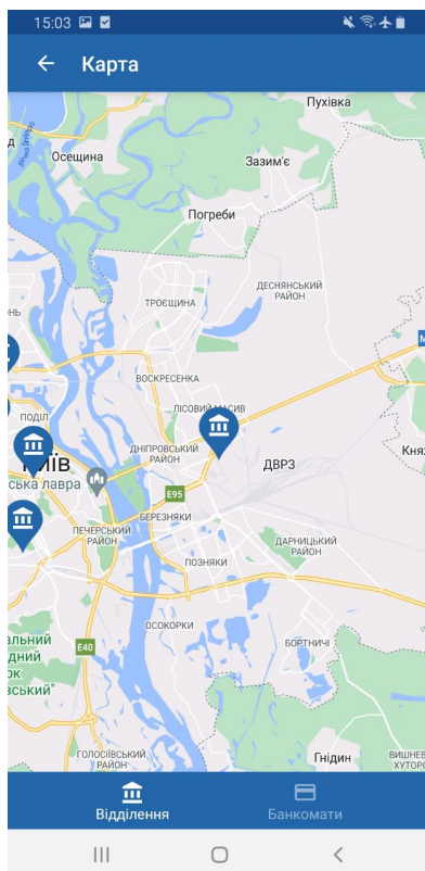
Рис. 13.1. Екран карти
