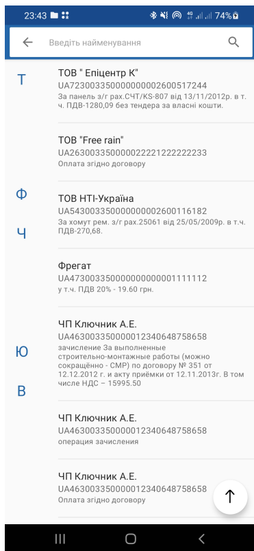
Рис. 6.4. Список одержувачів
