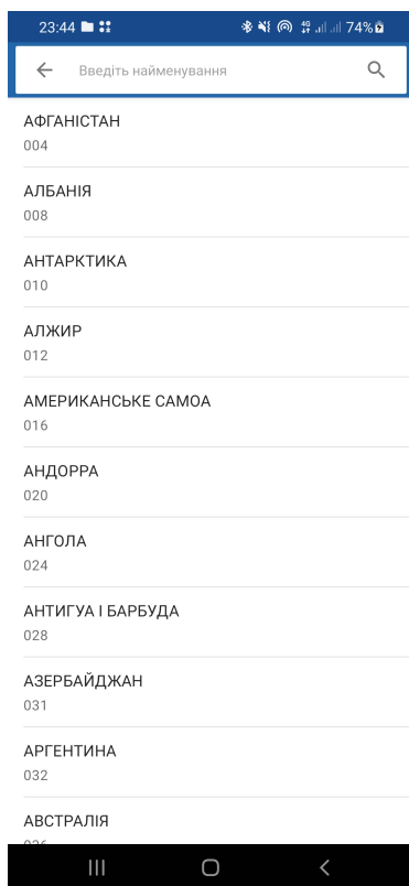
Рис. 6.5. Список країн
