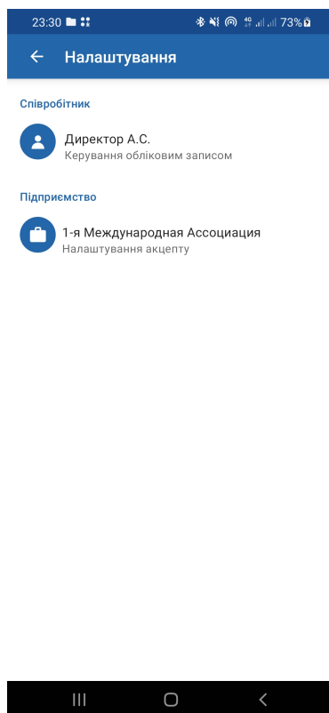
Рис. 4.2. Налаштування застосунку
